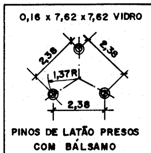
FIGURA 2 - PLACA DE VIDRO
