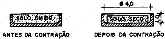
FIGURA 1 - CÁPSULA DE CONTRAÇÃO
