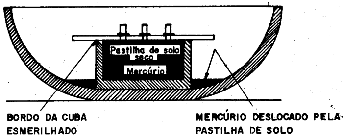
FIGURA 3 - APARELHO PARA DETERMINAÇÃO DOS FATORES DE CONTRAÇÃO DO SOLO
